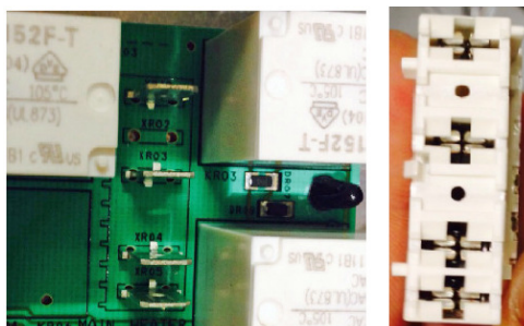
(3). Carte OVC3000 version simplifiée d'origine du four à dépanner et connecteur correspondant (4 broches).
