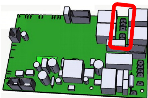
1. Emplacement des cosses et du connecteur sur la carte OVC3000.
