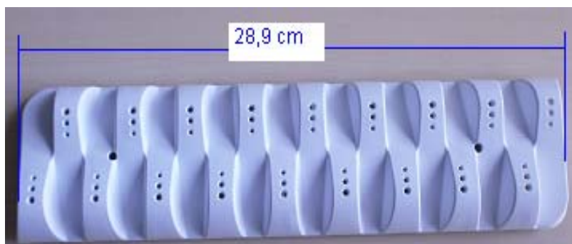
Photos et Dimensions réelles de l'aube
