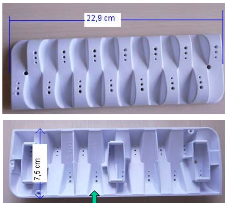
Photos et Dimensions réelles de l'aube
