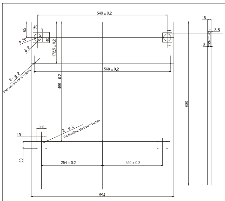
FIG. 3 Le panneau de la porte doit être placé comme décrit sur les dimensions illustrées sur ce dessin
